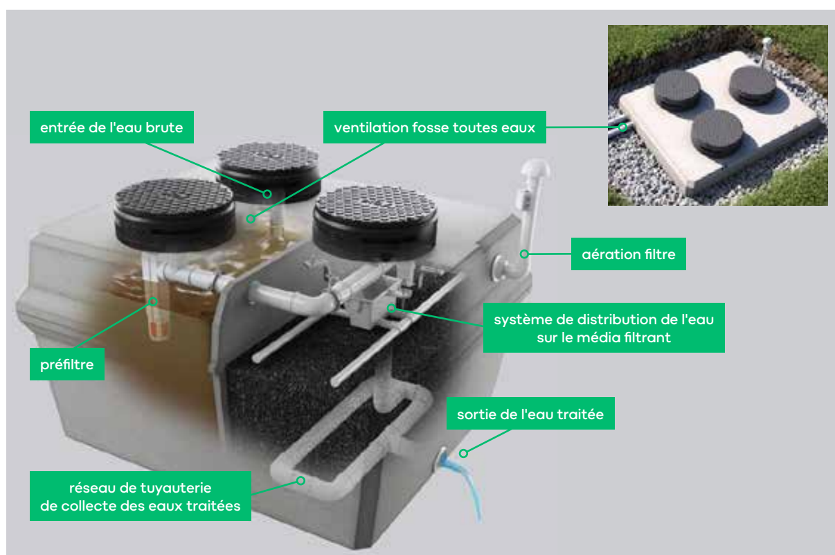
Fig-3 : principaux composants des x-perco® C-90 5 ou 6 EH monocuve
