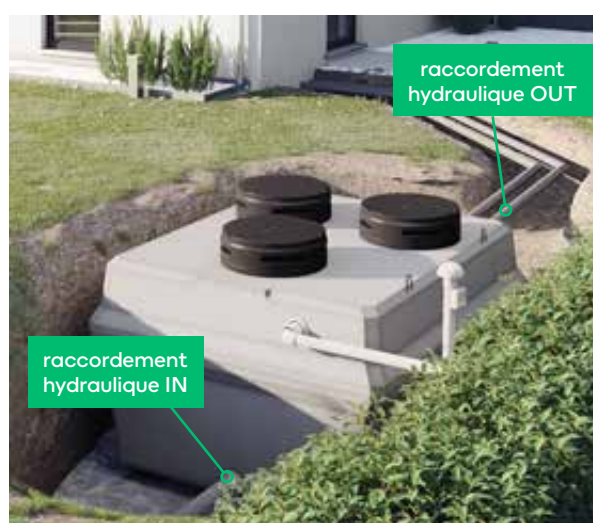
Fig-11 : raccordement hydraulique modèle 5 EH monocuve 6,5 m 3
