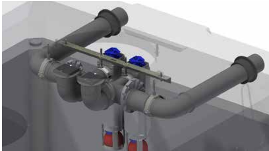
Fig-9 : exemple de dispositif de répartition dans une fosse toutes eaux C-90 6,5 m 3
