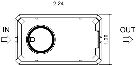
SEPTIC C-90 3 m³
